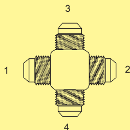
BF-2650 - Cross (1) (2) (3) (4) Male 45°
