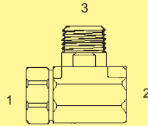
B-POL-2000 - Tee Check (1) (2) Fem. Inv. Flare (3) Male Pipe B-POL-2000
