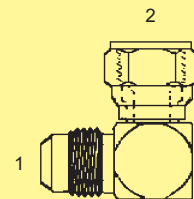
BF-6500 - 90° (1) Male 45° (2) 45° Fem. Swivel
