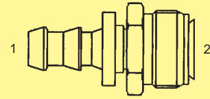
BPO-2290 - Str. (1) Hose Barb (2) Male Inv. Flare Swivel
