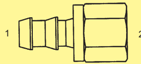
BPO-2274 - Str. (1) Hose Barb (2) Fem. Pipe Rigid
