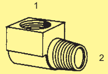
BIF-402 - 90° (1) Fem. Inv. Flare (2) Male Pipe
