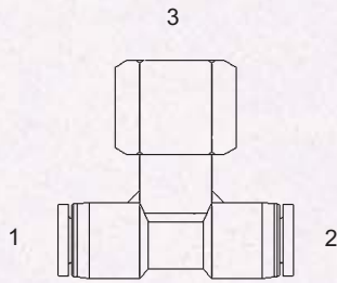
CPC-2602-S - Tee (1) (2) Tube (3) Fem. Pipe Swivel
