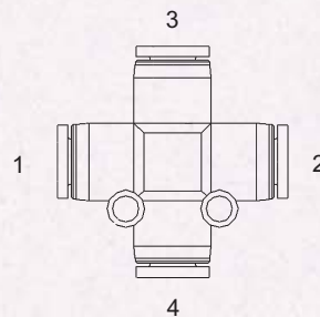
CPC-2650 - Cross (1) (2) (3) (4) Tube
