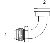
Y-1704-61 - 90° (1) Male 37° (2) O-Ring Flange Code 61
