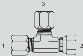
Y-FL-6602 - Tee (1) (3) Male Flareless (2) Fem. Flareless Swivel
