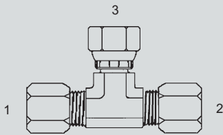
Y-FL-6600 - Tee (1) (2) Male Flareless (3) Fem. Flareless Swivel
