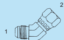
Y-SS-6502 - 45° (1) Male 37° (2) 37° Fem. Swivel
