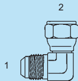
Y-SS-6500 - 90° (1) Male 37° (2) 37° Fem. Swivel
