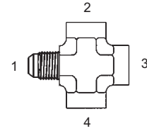
Y-2658-F - Tee (1) Male 37° (2) (3) (4) Fem. Pipe
