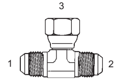
Y-6600-F - Tee (1) (2) Male 37° (3) 37° Fem. Swivel
