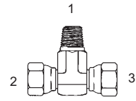
Y-1601-F - Tee (1) Male Pipe (2) (3) Fem. Pipe Swivel
