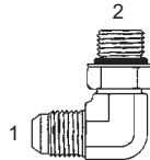
Y-6801-F-NWO - 90° (1) Male 37° (2) Adj. O-Ring
