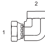
Y-6503-F - 90° (1) 37° Fem. Swivel (2) Fem. Pipe
