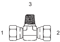
Y-6603-F - Tee (1) (2) 37° Fem. Swivel (3) Male Pipe
