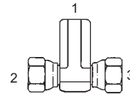
Y-1602-F - Tee (1) Fem. Pipe (2) (3) Fem. Pipe Swivel
