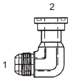
Y-1704-F-62 - 90° (1) Male 37° (2) O-Ring Flange Code 62
