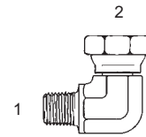
Y-1501-F - 90° (1) Male Pipe (2) Fem. Pipe Swivel
