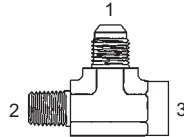
Y-2613-F - Tee (1) Male 37° (2) Male Pipe (3) Fem. Pipe
