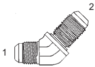
Y-2702-F - 45° (1) Male 37° (2) Bulkhead 37°
