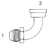
Y-1704-62 - 90° (1) Male 37° (2) O-Ring Flange Code 62
