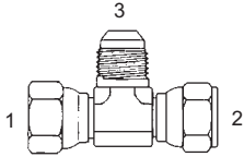
Y-6603-F - Tee (1) (2) 37° Fem. Swivel (3) Male 37°
