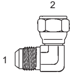
Y-6500-F - 90° (1) Male 37° (2) 37° Fem. Swivel
