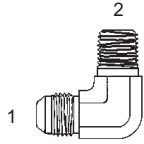
Y-2501-F - 90° (1) Male 37° (2) Male Pipe
