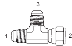
Y-6602-F - Tee (1) (3) Male 37° (2) 37° Fem. Swivel
