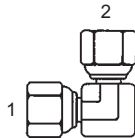
Y-6566-F - 90° (1) (2) 37° Fem. Swivel
