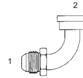
Y-1704-61 - 90° (1) Male 37° (2) O-Ring Flange Code 61
