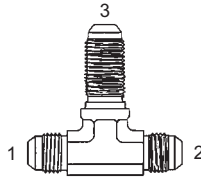
Y-2703-F - Tee (1) (2) Male 37° (3) Bulkhead 37°
