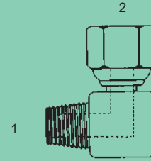
BPP-MBST-1501 - 90°
