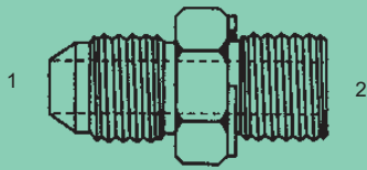
M-MJ-6400-DS - Str.
