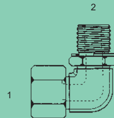
MFL-MB-6801-NWO - 90°
