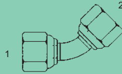
BPP-1514-L - 45° (1) (2) Fem. BPP Swivel - Long
