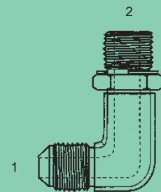
M-MJ-6801-L-NWO - 90°
