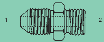
M-MJ-2404 - Str.
