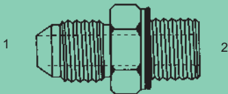
M-MJ-6400-WO - Str.
