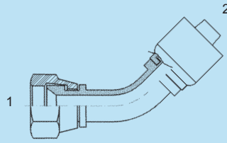
SSHE-88139 - 45° (1) Fem. 37° Swivel (2) Hose End
