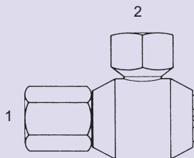
SLS-5504 - 90° (1) Fem. Pipe - Stem (2) Fem. Pipe - Barrel
